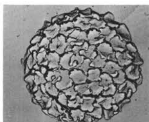
CALCAREOUS NANNOFOSSILS
