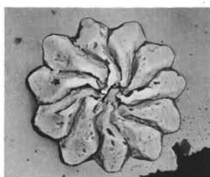
CALCAREOUS NANNOFOSSILS
